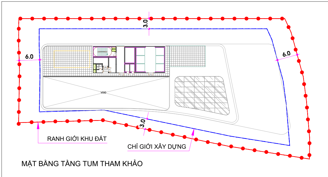
MẶT BẰNG TẦNG 39 THAM KHẢO
