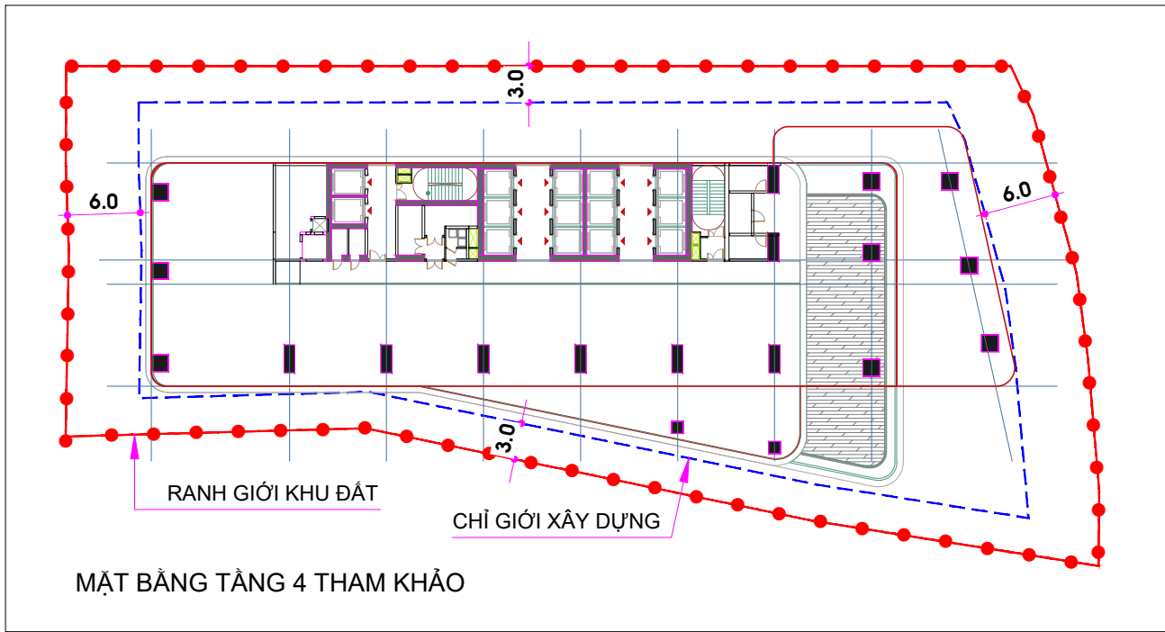
MẶT BẰNG TẦNG 2, 3 THAM KHẢO
