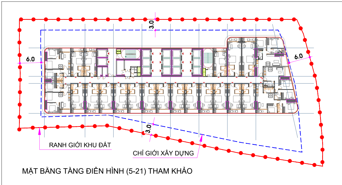
MẶT BẰNG TẦNG 4 THAM KHẢO
