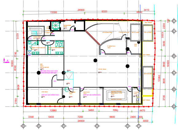
MẶT BẰNG TẦNG HẦM (THAM KHẢO)
