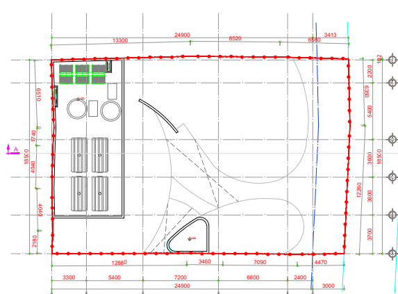
MẶT BẰNG TẦNG 10 (THAM KHẢO)
