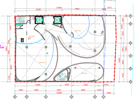
MẶT BẰNG TẦNG 2 (THAM KHẢO)
