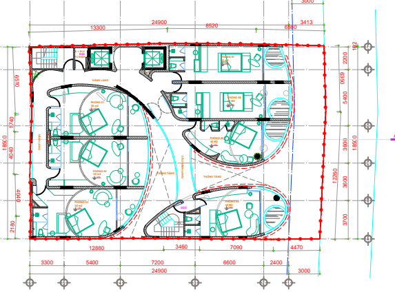
MẶT BẰNG TẦNG 3 (THAM KHẢO)
