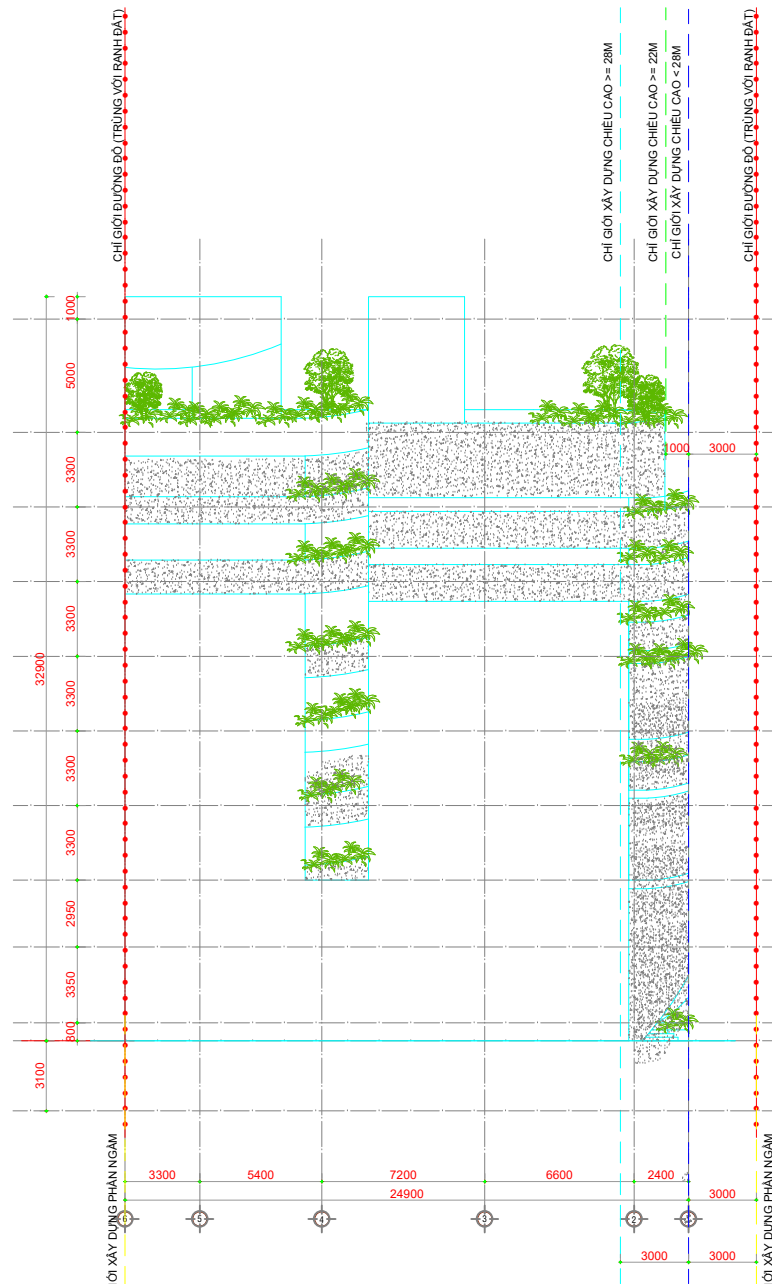
MẶT ĐỨNG TRỤC 6-1(THAM KHẢO)
