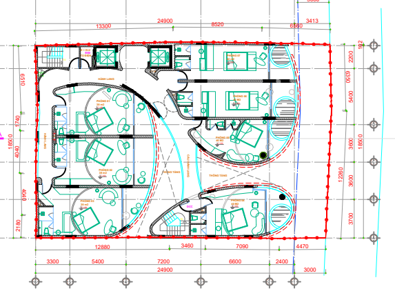
MẶT BẰNG TẦNG 7 (THAM KHẢO)
