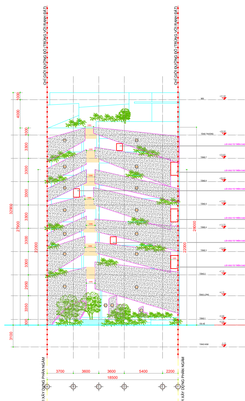
MẶT ĐỨNG CHỈNH (THAM KHẢO)
