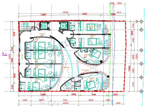
MẶT BẰNG TẦNG 8 (THAM KHẢO)
