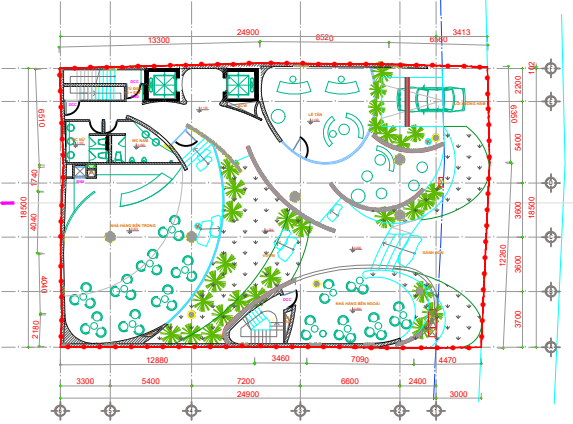
MẶT BẰNG TẦNG 1 (THAM KHẢO)
