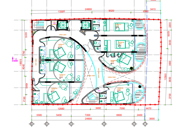
MẶT BẰNG TẦNG 6 (THAM KHẢO)
